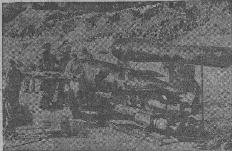
En Norteamérica comenzaron a construir el "V-4" con arreglo al modelo alemán. Los primeros ensayos se han realizado, al parecer, con éxito. La foto ha sido hecha en una pista de despegue (Orbis-Foto)
