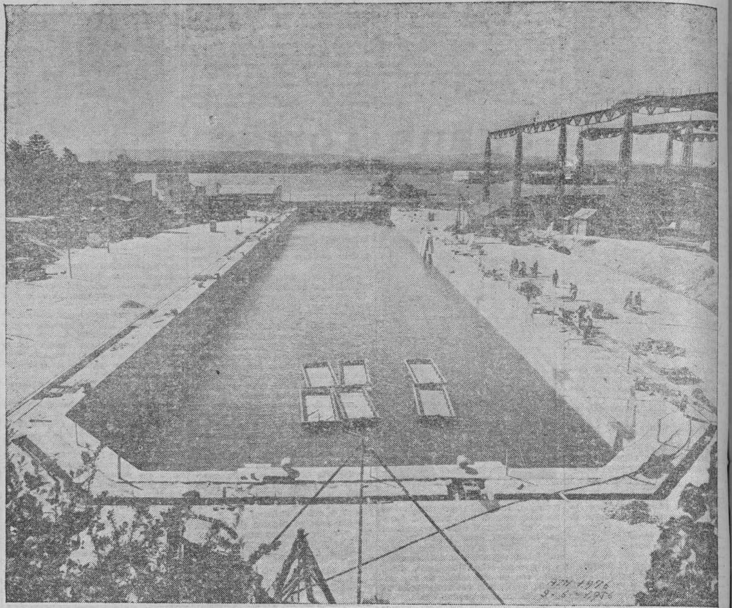
Maqueta de los Astilleros y Talleres del Noroeste S. A. en la que ya figuran las obras de ampliación.
