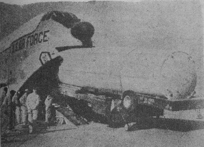
Del "almacén" de un avión militar norteamericano sale el cuerpo de un "Thor", capaz de transportar dos mil kilogramos una cabeza nuclear. Se presenta en el Salón Aero-náutico de París
