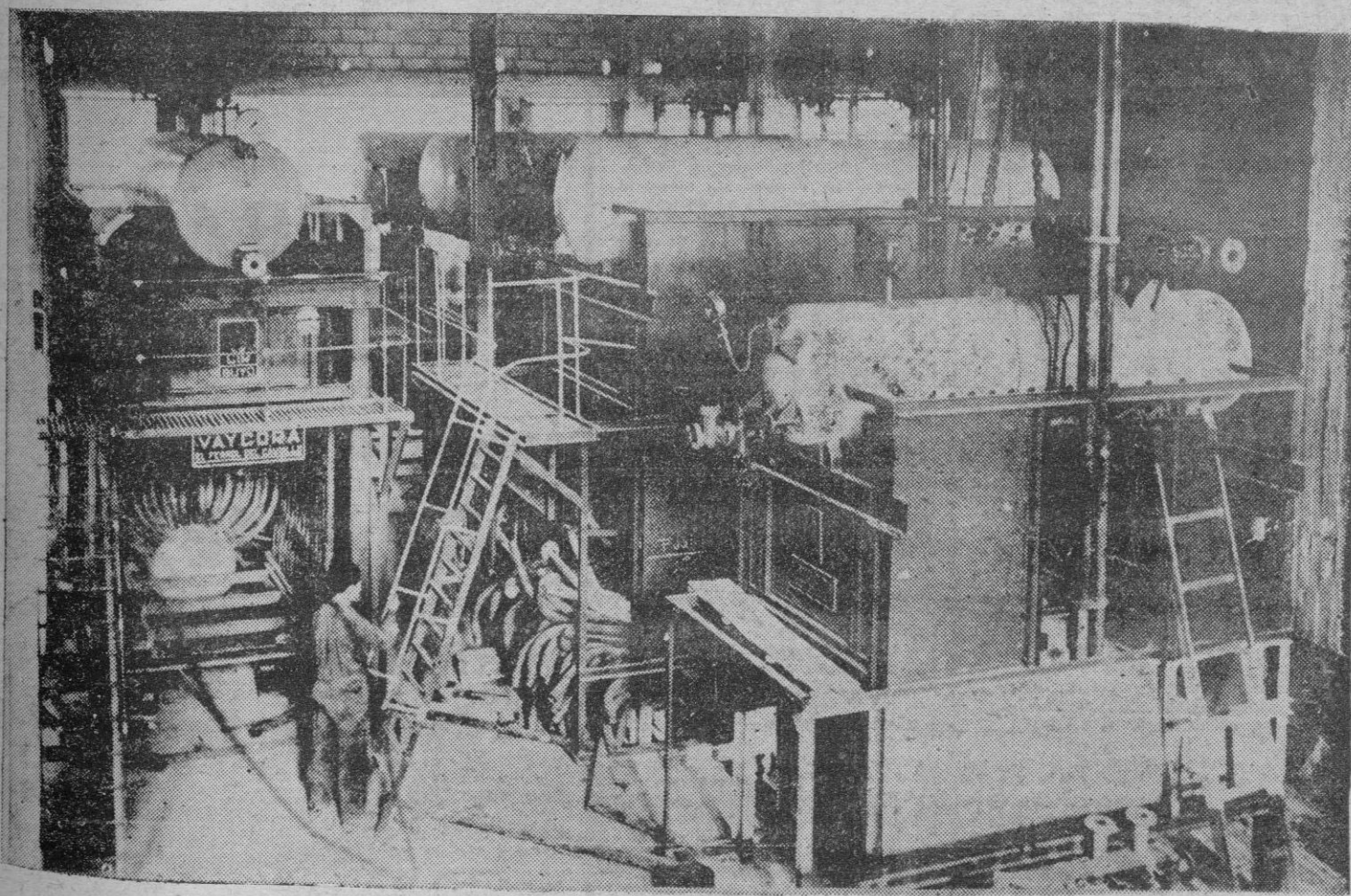
Vista parcial de una de nuestras naves de montaje con cinco calderas en período de construcción
