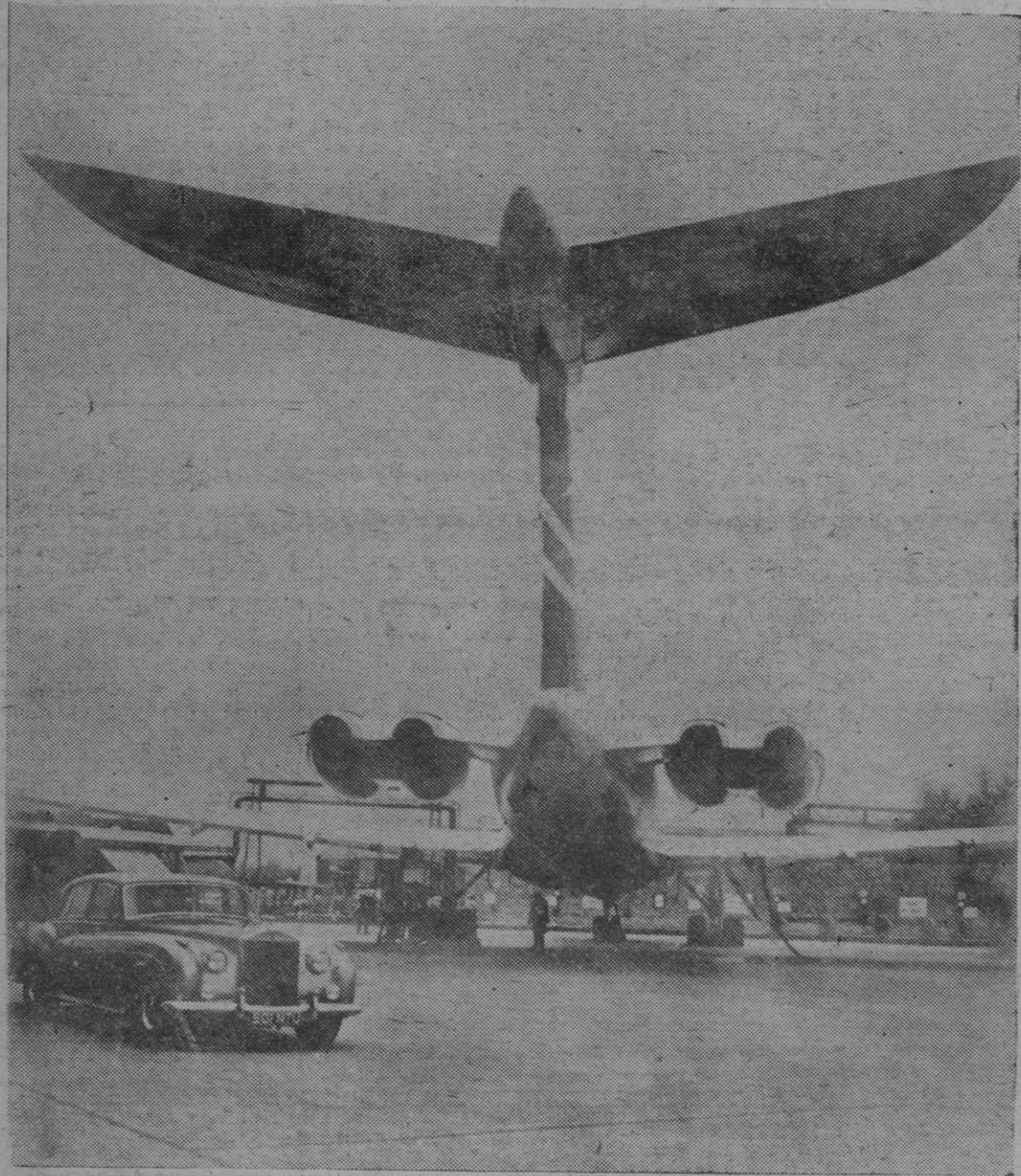
Una foto del VC-10, avión a reacción, en la que se aprecia su elevada cola y los cuatro motores Rolls-Royce Conway
