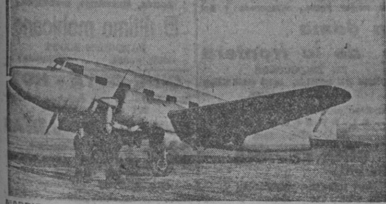
MADRID.—He aquí el avión comercial "Alcotán", totalmente construido en España y cuya primer prueba ha presenciado el Ministro del Aire en el aeródromo de Getafe
