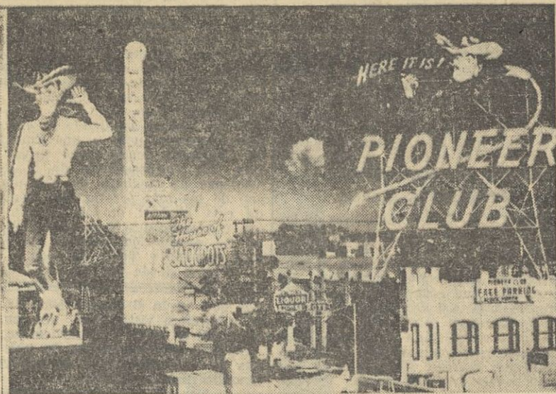
LAS VEGAS (NEVADA).—He aquí una curiosa fotografía de la ciudad, con sus anuncios luminosos, que sirven de marco a la explosión atómica representada por esta nubecilla, ya típica, que se perfila en el horizonte. (Foto CIFRA).
