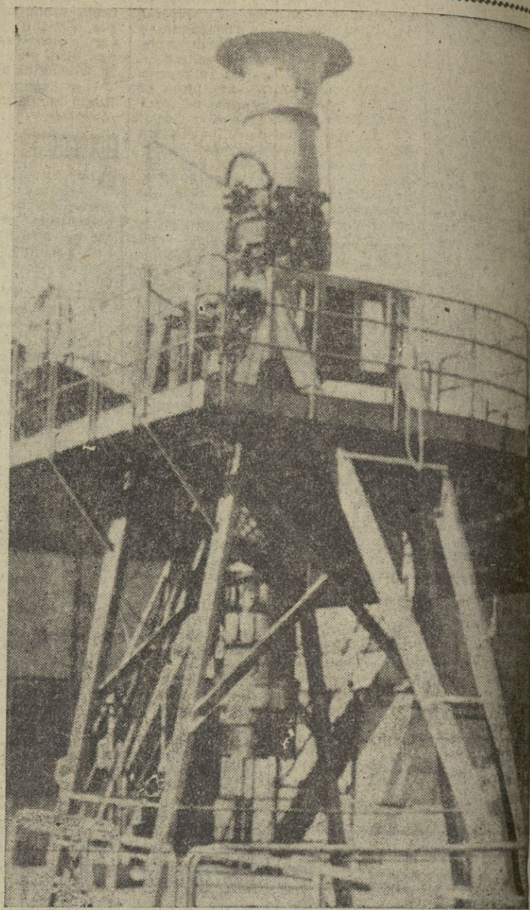
Esta telefoto muestra el aparato construido en Francia para investigar los despegues verticales de los aviones (Foto A. Pi)
