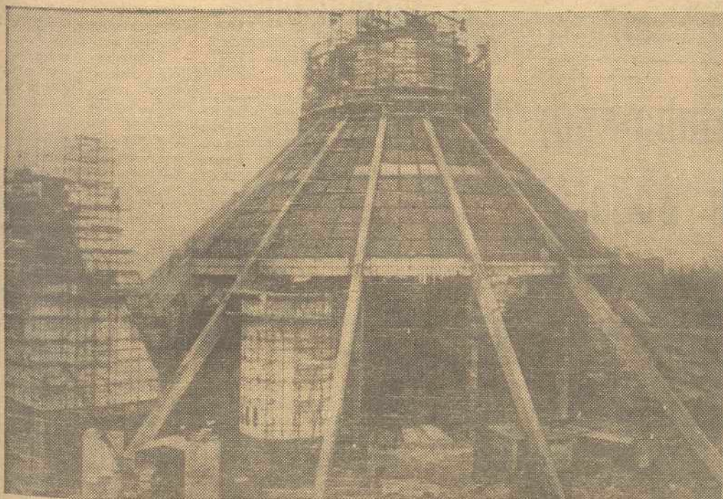
Un aspecto de la erección de la base cónica de la nueva catedral católica de Brownlow Hill (Liverpool), que será construida con hormigón reforzado en su mayor parte. El cono central se prolongará en una torre cuyos campanarios quedarán a noventa y nueve metros de altura. La obra finalizará en 1968. — (Foto AP-LOGOS).
