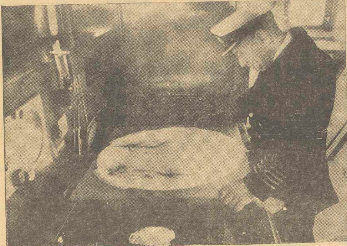
Un oficial de derrota examina el estuario del Támesis a través de un instrumento radárico "Kelvin Hughes Photoplot"
