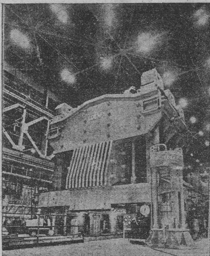
Esta prensa, cuya presión iguala al peso de un portaviones de 50.000 toneladas, ha sido montada en los Estados Unidos para la construcción de piezas fundamentales con destino a los nuevos "Superconstellation". La altura de la prensa es la de un edificio de diez pisos y está sustentada por seis columnas de 300 toneladas de peso cada una.
