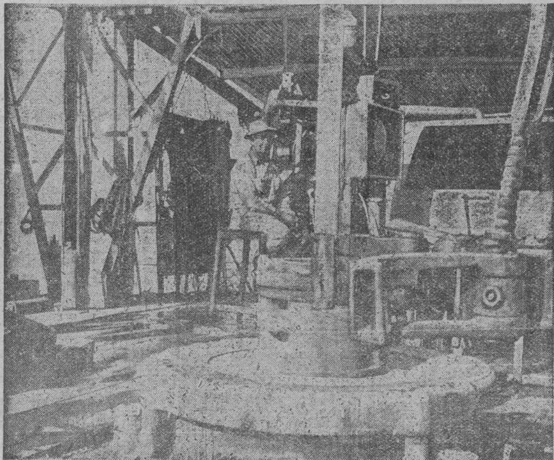
Un técnico atiende el trabajo de las perforadoras en un pozo petrolífero del Oriente Medio
