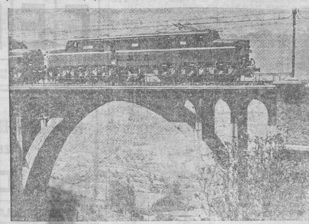
Paso de dos locomotoras de la serie 7.700 por el puente de Valdeleón, en la línea de León a Gijón, que como la mayoría de estas obras cambió el acero por el hormigón (parte inferior) sin interrumpir la circulación de trenes.—(De la revista TRENES)
