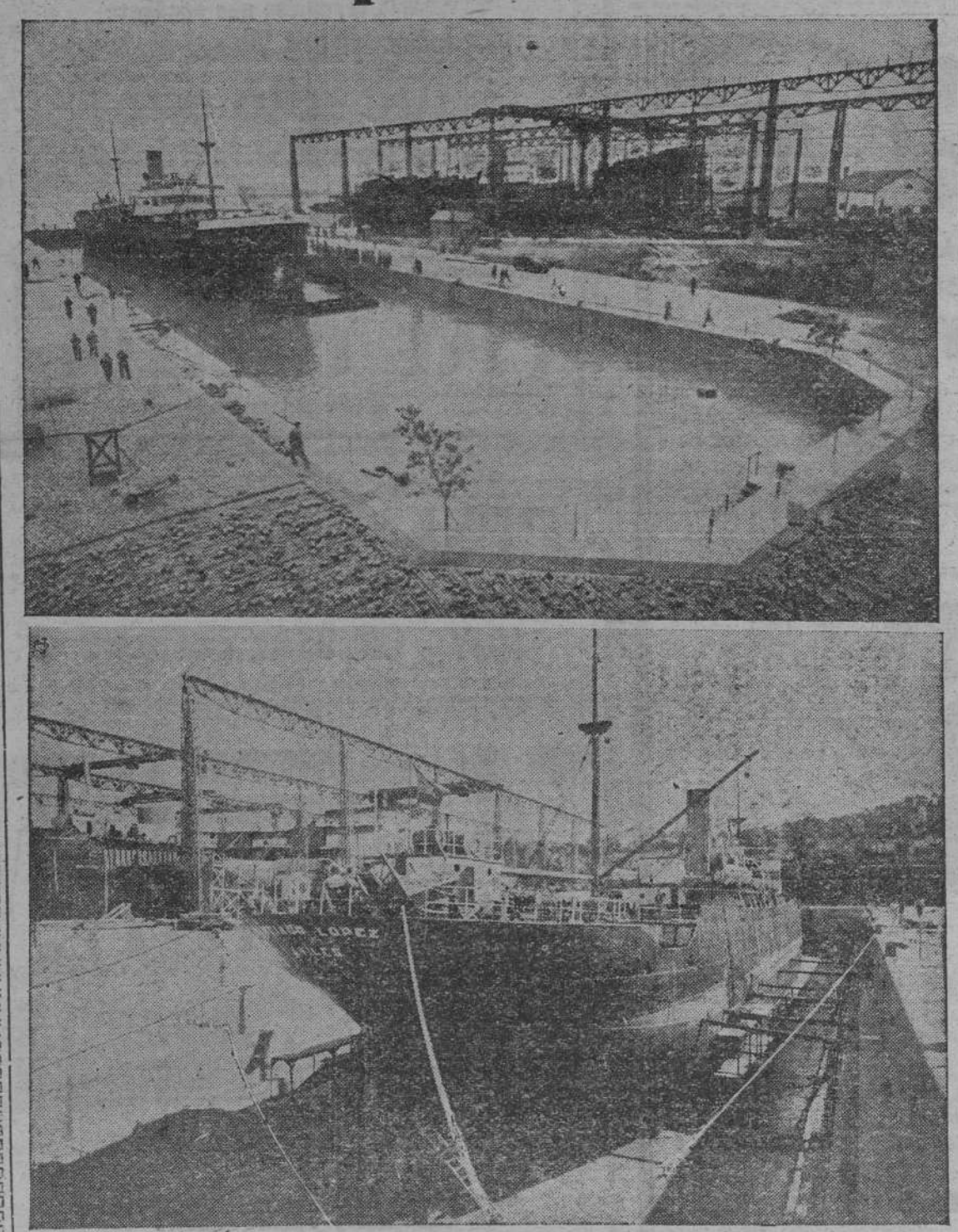
El martes ha sido inaugurado en Perito (El Ferrol del Caudillo) un nuevo dique de la Empresa ASTANO capaz para barcos de 3.000 toneladas. Nuestra información gráfica ofrece un aspecto de la importante obra y otro plano en el que vemos al barco "Santiago López" totalmente en seco dentro del magnífico dique. —(Foto Bernardina Suardes)
