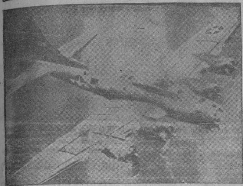
Una Fortaleza Volante B-17, americana, en vuelo. La torreta inferior va provista de dos cañones de calibre 50, y el avión pesa unos 30.000 kilogramos. Su carga de bombas es de 3.000 kilogramos, y su velocidad de unos 450 kilómetros por hora. (Foto recibida por radio).
