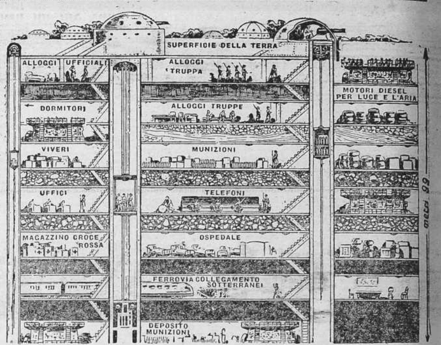
Gráfico de una sección de la línea Maginot, con el sistema completo de comunicaciones. La línea fortificada a flor de tierra cerca de Alemania es una serie de torres blindadas perfectamente artilladas
