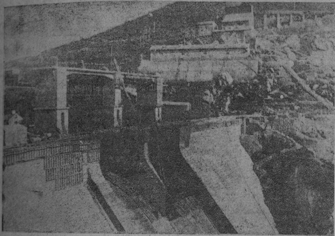
La presa de Liño sobre el río Tambre, y que reforzará grandemente las disponibilidades de energía de la Sociedad General Gallega de Electricidad. (Foto Arturo).
