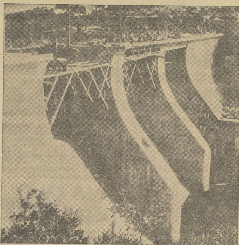
Presas del pantano de Rosquito, sobre el Tietar, de 24 metros de altura y 72 de longitud, que podrá embalsar 84 millones de metros cúbicos de agua, lo que permitirá un riego de 17.000 hectáreas de las vegas de la Vera y Navalmaral de la Mata. El salto de agua generará 17 millones de kilovatios-hora al año. Dicho pantano, fué inaugurado en días pasados por el Ministro de Obras Públicas
