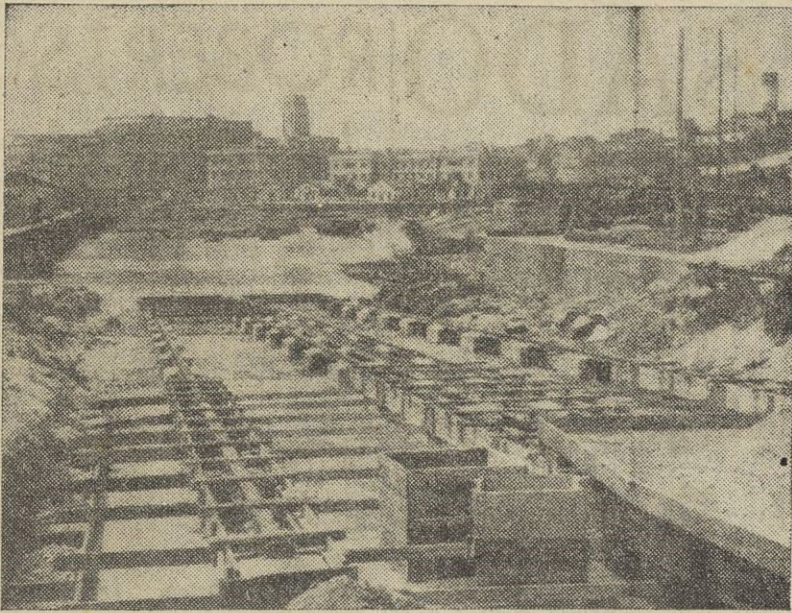
Estos días se está procediendo a la instalación del carro mecánico en el varadero para barcos pesqueros construido en el Parrote. En la foto, un aspecto de las obras
