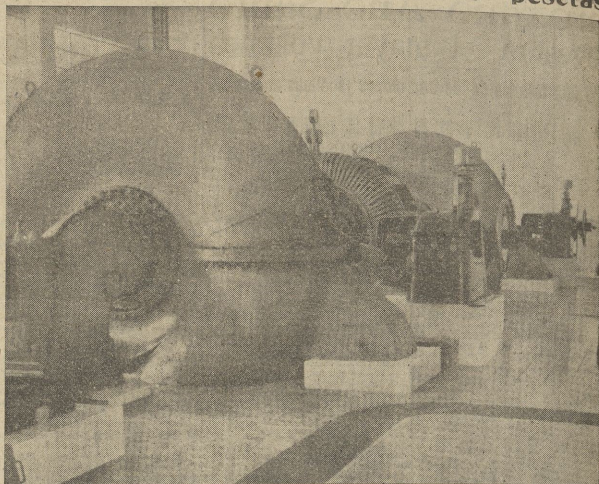
Planta de una central hidroeléctrica de 60.000 H. P. de potencia, semejante a la que se instalará en la Capela
