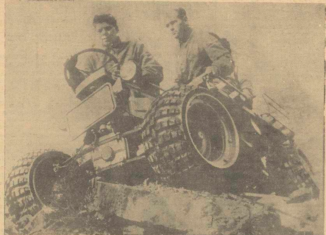
El «carro de fuerza», un vehículo de cuatro ruedas que goza de gran movilidad en todo terreno, cuenta con una gran capacidad de carga, reducido peso y manejo sencillo durante su presentación por el Centro Alemán de Protección Civil de Bonn. Está calificado como el más perfecto de los utilizados en catástrofes como terremotos, inundaciones, derrumbamientos, bombardeos, etc.
