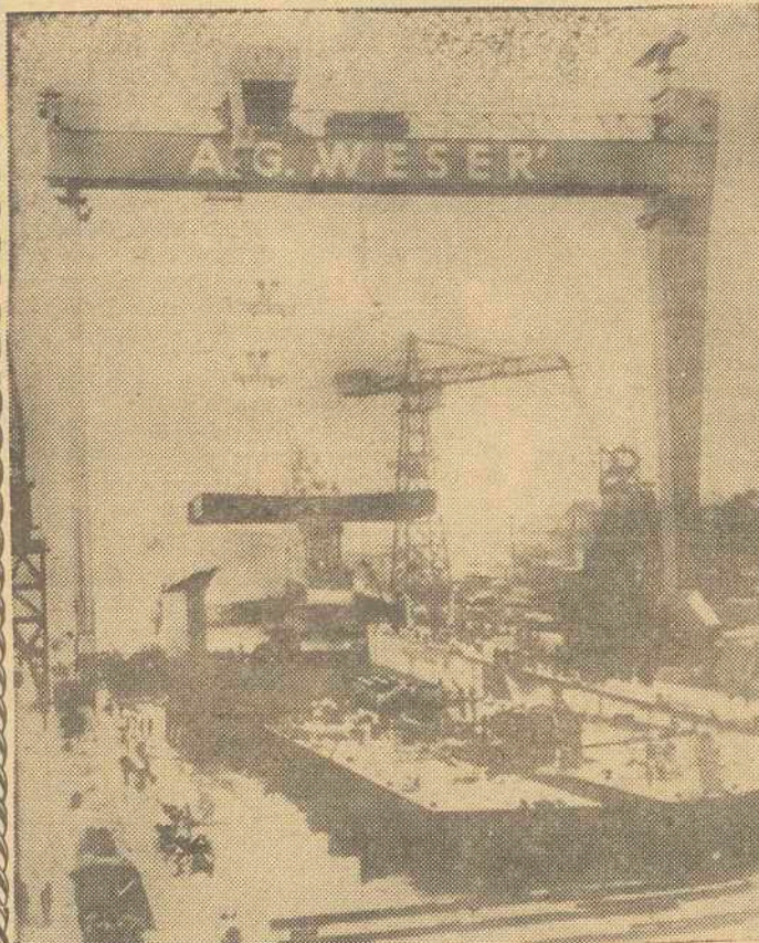
En los astilleros del puerto alemán de Bremen se levanta la grúa más grande del mundo. Con 74 metros de altura y 65 de anchura entre los dos carriles por los que se mueve, puede elevar cargas de hasta 500 toneladas y manejarlas con exactitud de milímetros. — (FOTOFIEL)
