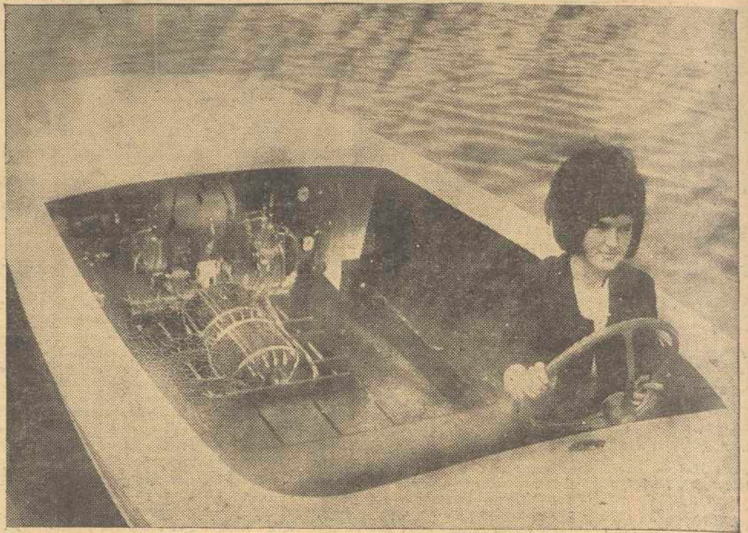
MUNICH.— Con cinco personas a bordo esta lancha automóvil desarrolla una velocidad de siete kilómetros por hora. Esto no sería nada de importancia si no se tratara de admirar un sistema de propulsión completamente nuevo. Células de combustible, que en lugar de nocivos gases de escape de mal olor no segregan sino agua purísima, accionan un electro-motor prácticamente sin ruido. Hombres de ciencia de la Alemania Occidental desarrollaron láminas delgadas de combustible, de 30 centímetros de altura, que se pueden apilar formando columnas para conseguir tensiones más altas. A cada célula se aporta a un lado gas de
