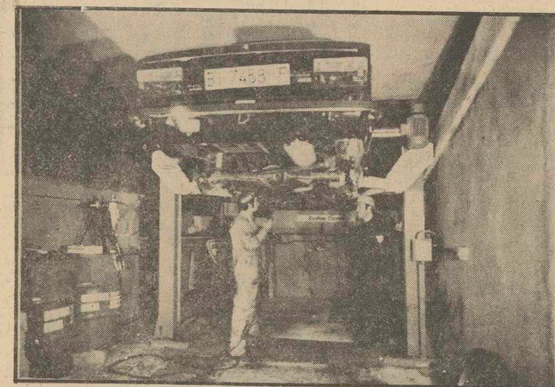
Inyección del producto DINITROL ML en una viga del chasis
