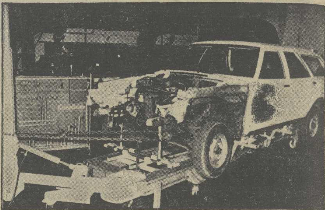
Esta máquina, fabricada en Suecia y capaz de desarrollar una fuerza de tracción de hasta diez toneladas, puede reparar rápidamente coches accidentados que hasta ahora eran considerados irreparables. Aquí la vemos en acción, en un taller de Inglaterra, "alisando" un automóvil totalmente abollado. — (FOTOFIEL - TOPIX)
