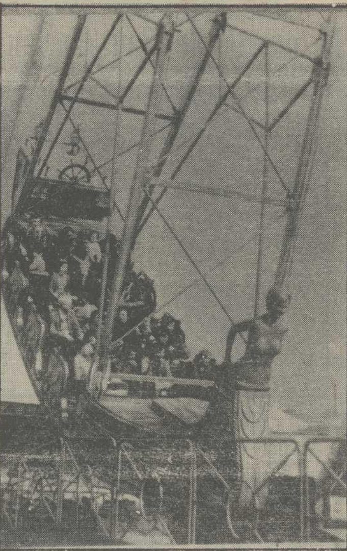
En los talleres Pflaum, de Neue Elm (República Federal de Alemania), ha sido construida esta gran góndola columpio, de 9,80 metros de eslora, que pronto se ha convertido en una de las atracciones principales de las ferias alemanas. Está accionada electrónicamente y antes de ser autorizada fue sometida durante tres años a diferentes pruebas de seguridad. — (Foto DaD/Pflaum)
