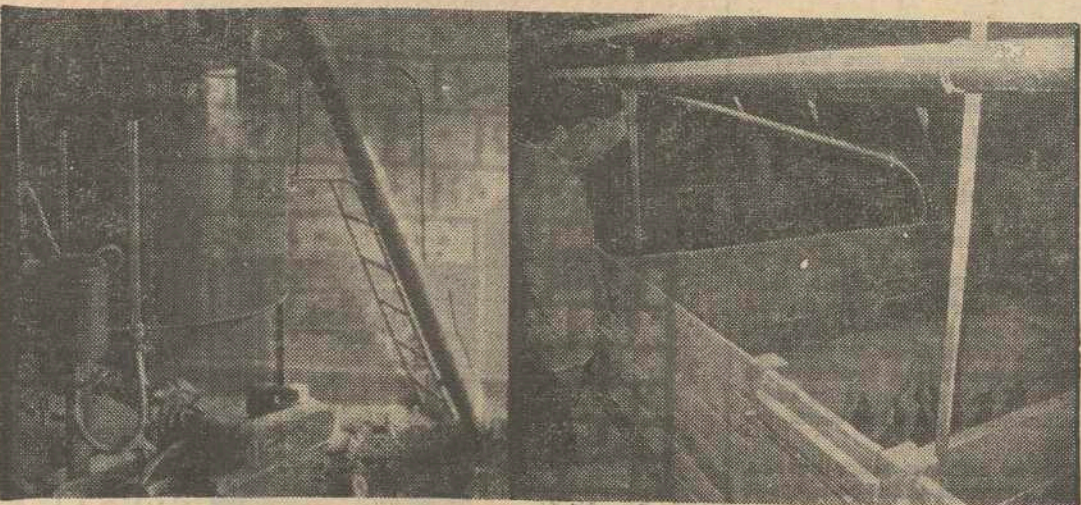
A la izquierda, máquina de papilla de mil litros. La bomba, debajo del depósito, efectúa la mezcla de la papilla y también envía ésta hacia las pilas de las cerdas. A la derecha, las pocilgas son atravesadas por los dos conductos de traida y retorno de la papilla. Un operario, abriendo una compuerta, vierte el alimento en cada pila
