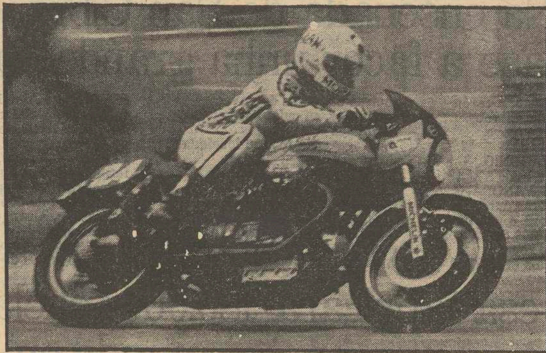
Carlos Morante, pilotando la moto Guzzi modelo Le Mans 850, en el circuito de Pocomac, en La Coruña, con la que venció en las doce horas de resistencia, haciendo equipo con Pérez Rubio. Esta moto presenta estas características: motor bicilindro kilos y velocidad máxima 210 Km./H. de potencia a 7.600 r. p. m. Peso 19drico en uve, de cuatro tiempos y 844 c. c., 90 CV
