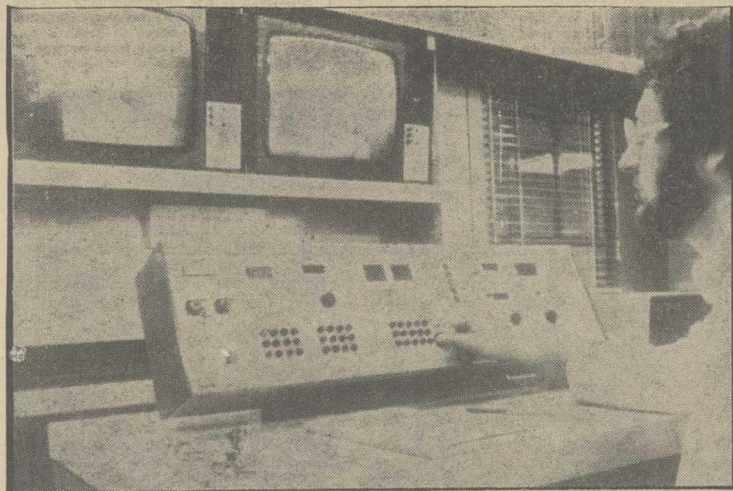
Este es el panel de mando del betatrón 500 A, aparato desarrollado en el Instituto Central de Investigación del Cáncer de Berlín Oriental, desde donde se regula y controla los procesos radiológicos (densidad y espesor de los rayos). Largos años de investigación con todo tipo de radiación (rayos X, radiación de electrones o de neutrones) han posibilitado a los científicos establecer la dosis óptima de radiación para un enfermo y garantizarla mediante este betatrón. —(FOTOFIEL)
