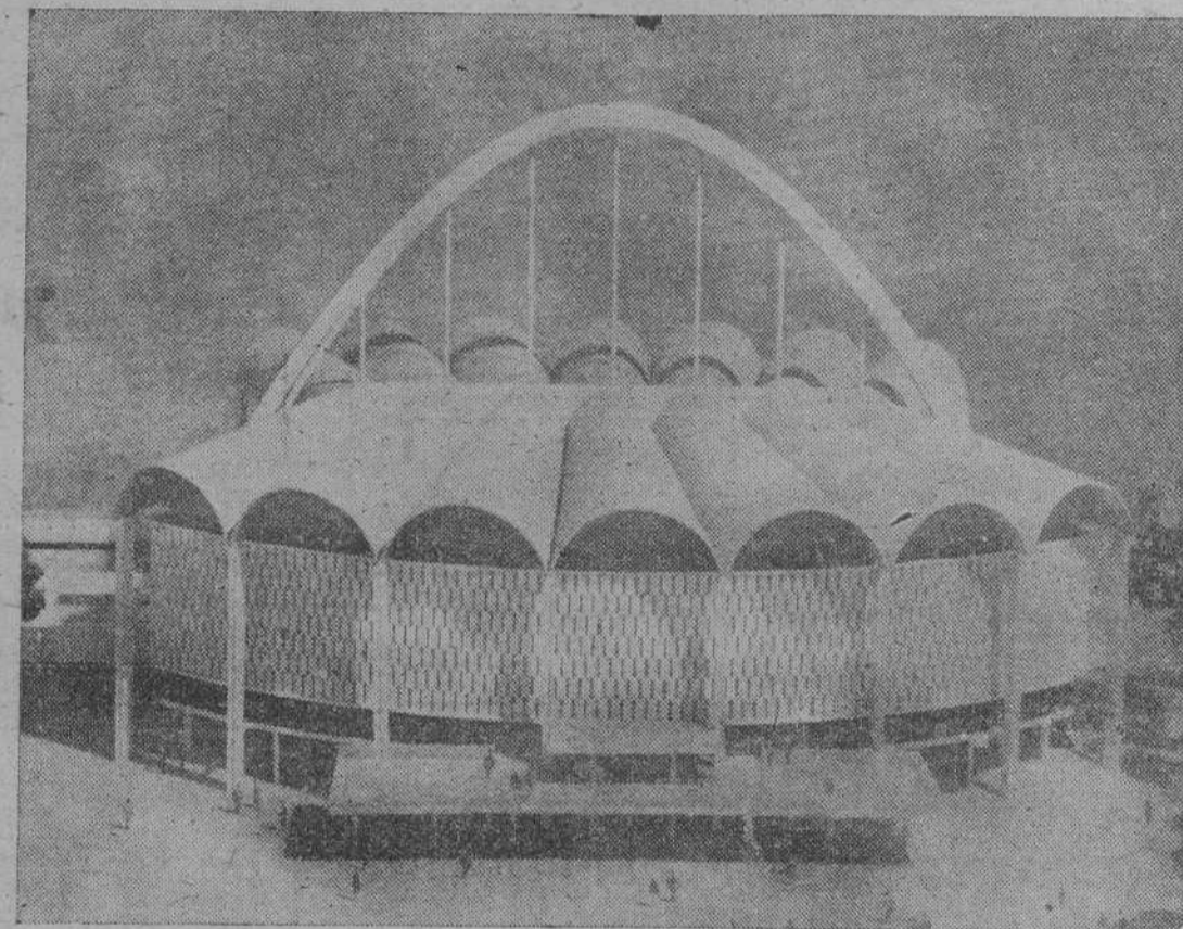
Proyecto de "Auditorium" para Tallahassee, (Florida, EE. UU.), con techo tubular, sostenido por un arco de hormigón. El interior queda sin columnas para no impedir la visión a los espectadores. Arquitecto Walter Gropius.
