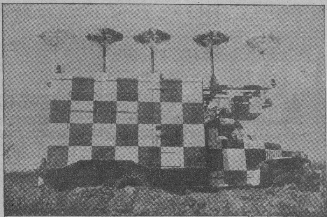
Igual que cualquier camión, pero con aspecto de tablero de damas. Las antenas del "I.L.S.", de forma caprichosa, aparecen en volutas en zigzag para preservarlas de la humedad. (Foto Arturo)
