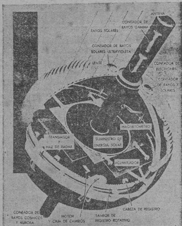
Un esquema del proyecto del satélite americano
