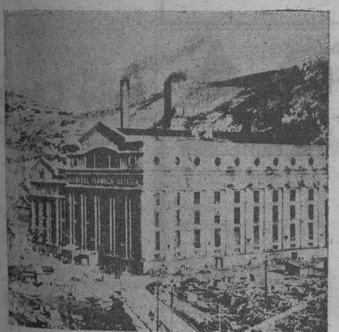
La nueva central eléctrica de Aliaga. Consta de tres grupos generadores, cuya potencia total, a pleno rendimiento, es de cuarenta y siete mil kilovatios. — (Cifra)
