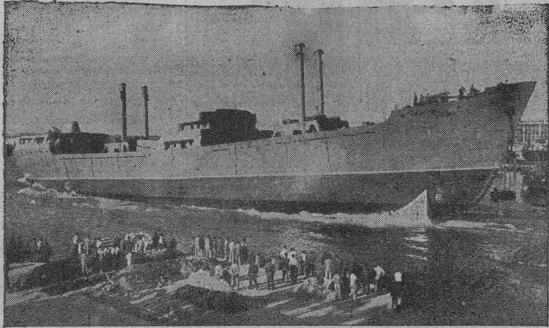
Momento de abandonar la grada el buque "Río Umla". Construido por "Arsilleros y Talleres del Noroeste, Sociedad Anónima, ASTANO", de El Ferrol del Caudillo. (Foto Bernardino González)
