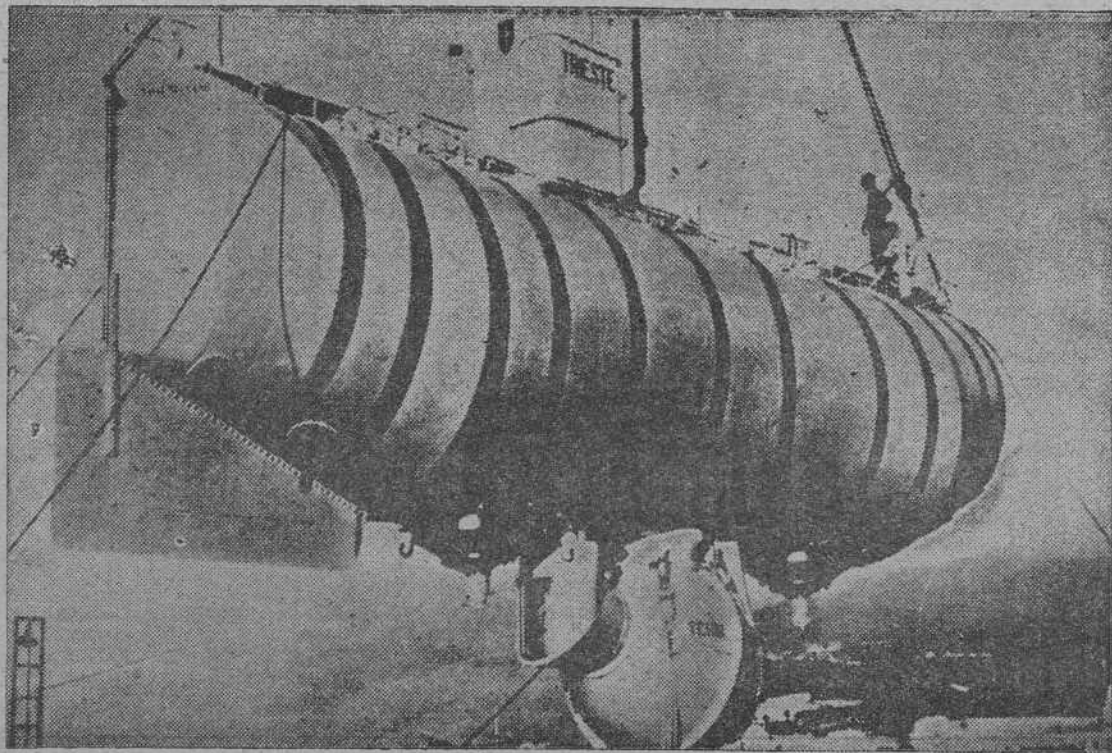
El batiscavo "Trieste", construido en la ciudad de su nombre, por encargo de la Marina norteamericana, según diseño de los profesores Piccard, padre e hijo.
