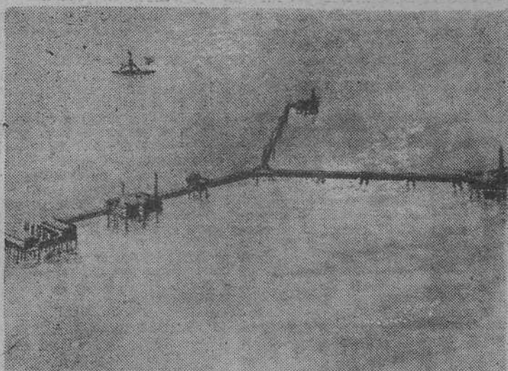
La gigantesca estructura de acero tiene forma de "Y" y costará unos 30 millones de dólares. Se apoya en pilares de acero de 75 metros de alto que reposan en el fondo y elevan el conjunto a 18 metros sobre el mar.
