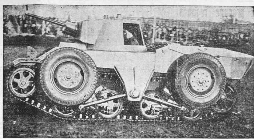
Este tanque puede rodar indistintamente sobre las orugas o sobre las ruedas, por simple manejo en el interior, ejecutado en 18 segundos. La velocidad sobre las orugas es de 40 kilómetros por hora, y sobre las ruedas de 75 kilómetros. Van tres hombres en el interior. Una ametralladora y un cañón, son su armamento
