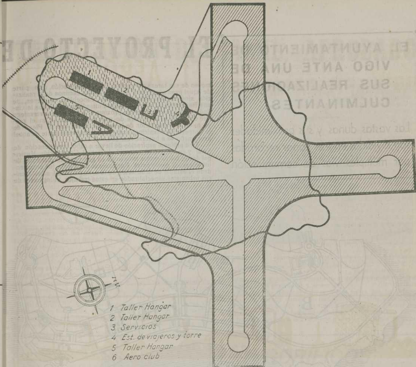
Plano del Aeropuerto de Peinador según el proyecto en curso de realización. En él se indica, con su trazo curvo y fino, el área ya explanada, así como la pista de despegue construida.
