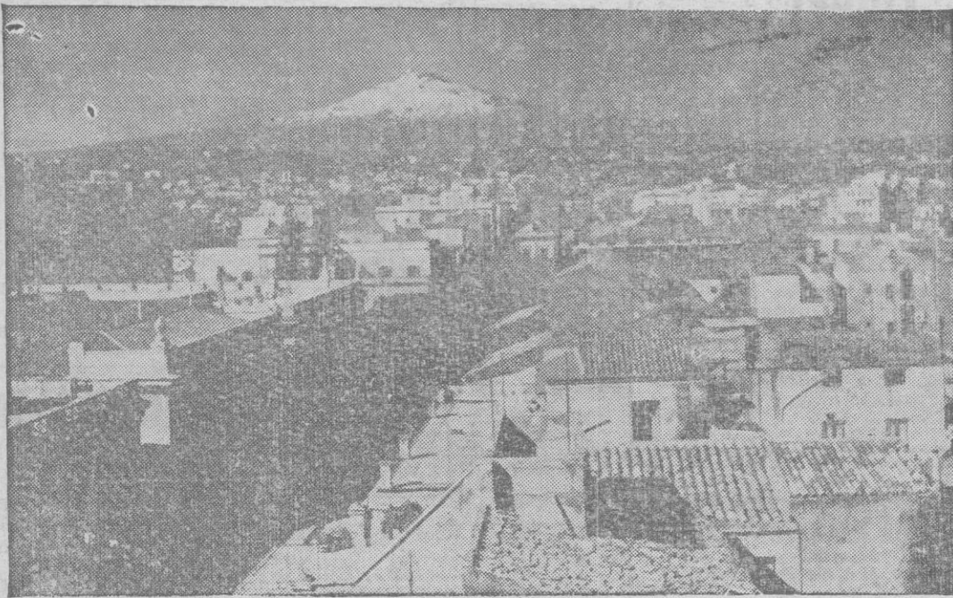
Vista general de Catania (Sicilia) al fondo, el Etna
