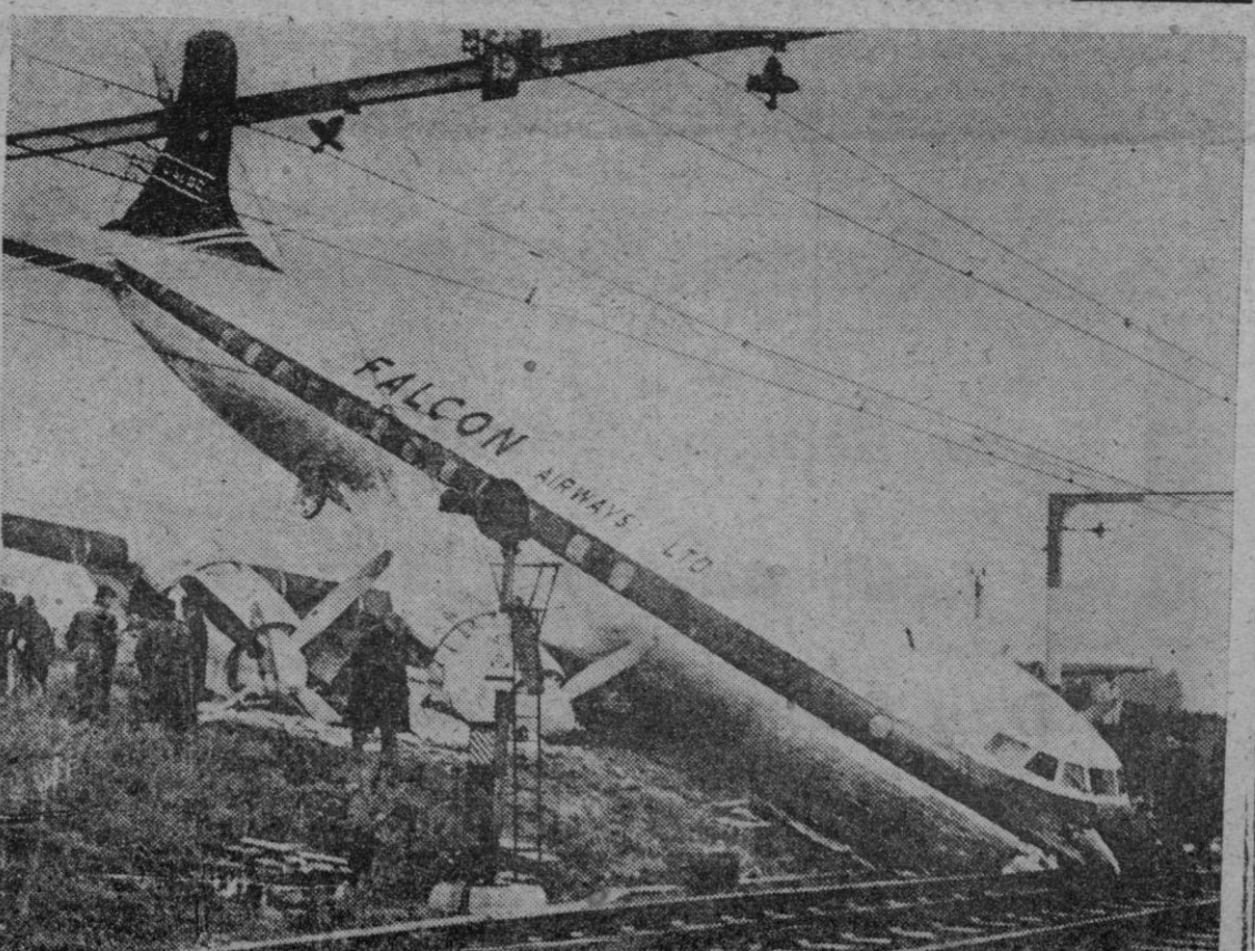
Un avión británico, en las cercanías de Southend, aterrizó de esta manera sobre las vías del tren cuando trataba de hacerlo en el vecino aeropuerto. No chocó con los cables de alta tensión y tampoco pasaba entonces ningún tren. De las 76 personas que viajaban a bordo, solamente cuatro hubieron de ser hospitalizadas por pequeñas confusiones recibidas.
