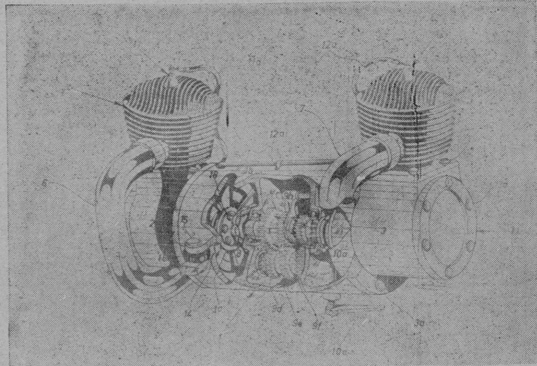
Vista general del motor de dos tiempos creado por el señor R. Pereiro, para coche utilitario
