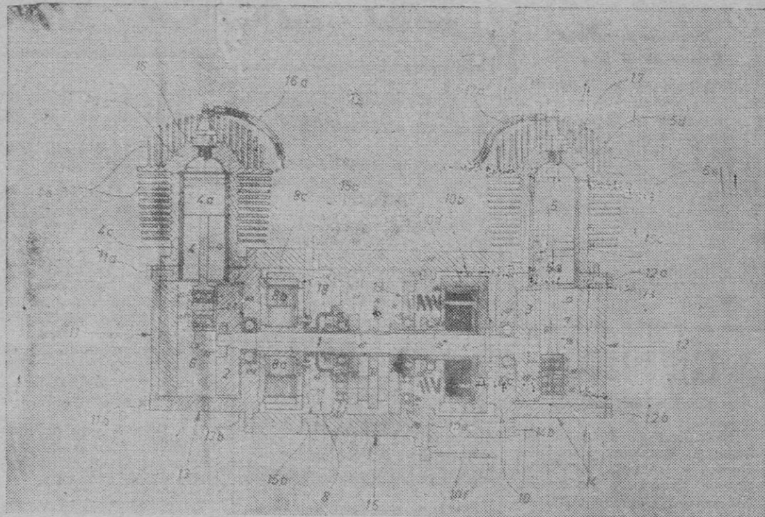
Diseño del motor de dos tiempos para coche utilitario, inventado por don José R. Pereiro.
