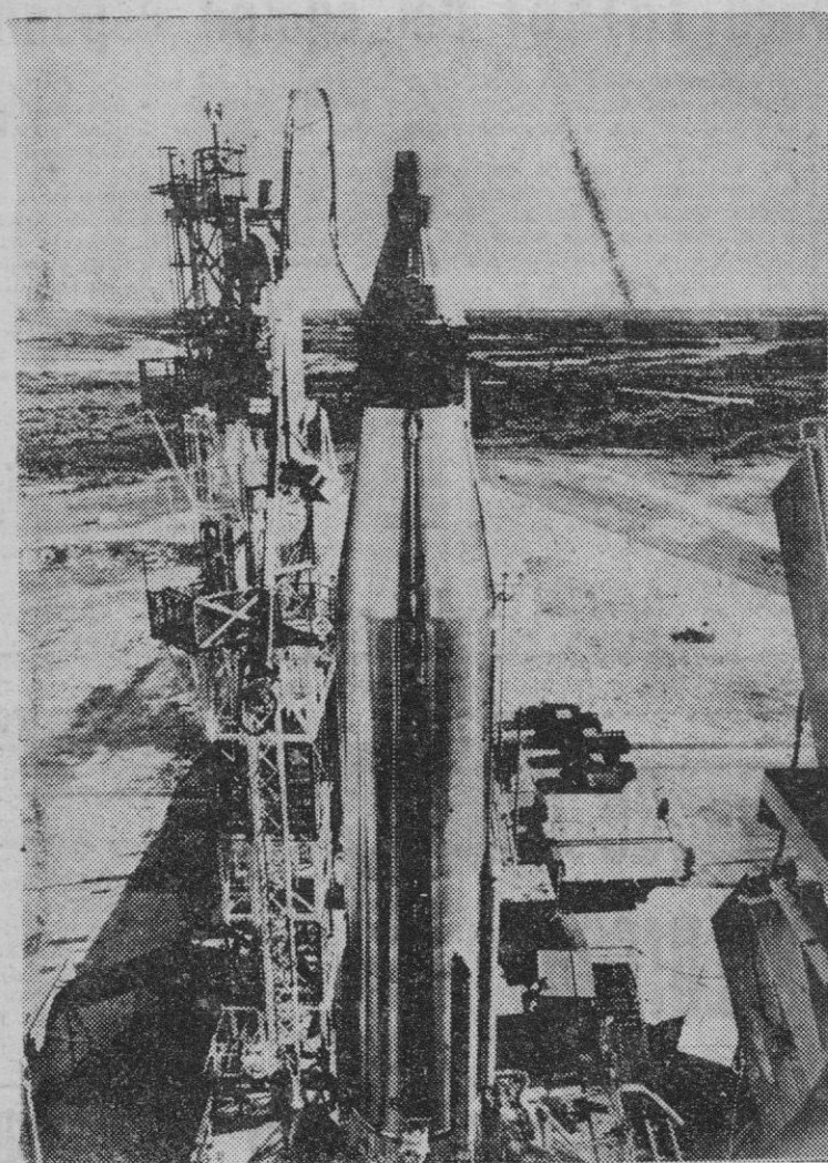
Un proyectil "Atlas", poco antes de ser lanzado desde la base de Cabo Cañaveral. La altura del proyectil desde la base de la unidad propulsora hasta lo más alto de la cápsula es de veintiséis metros (Foto Europa Press)
