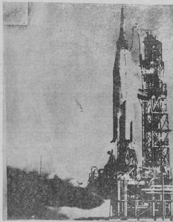
El "Atlas" con la cápsula "Mercury" y la torreta de salvamento, dispuesto para la prueba final
