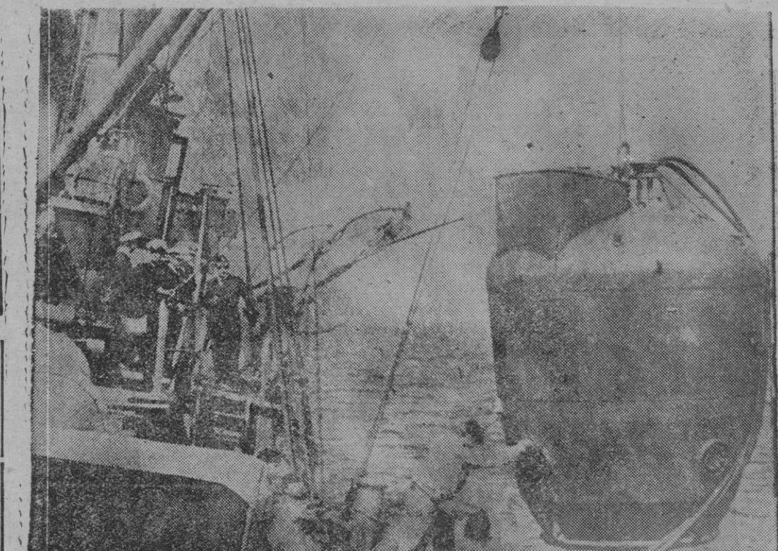
LUELSMINDE. -- En las costas de Jutianda, oficiales de las Marinas sueca y danesa están probando en estos días un aparato de invención norteamericana para el salvamento de las tripulaciones de los submarinos hundidos. El depósito aquí fotografiado, que, dirigido por un hombre, desciende hasta la escotilla del sumergible, tiene capacidad para subir a siete hombres en cada viaje hasta la superficie.
