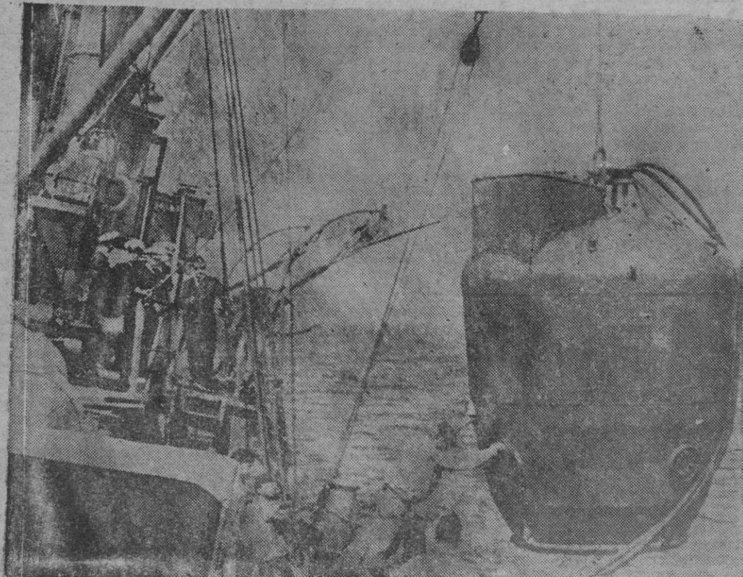
LUELSMINDE. En las costas de Jutianda, oficiales de las Marinas sueca y danesa están probando en estos días un aparato de invención norteamericana para el salvamento de las tripulaciones de los submarinos hundidos. El depósito aquí fotografiado, que, dirigido por un hombre, desciende hasta la escotilla del sumergible, tiene capacidad para subir a siete hombres en cada viaje hasta la superficie.
