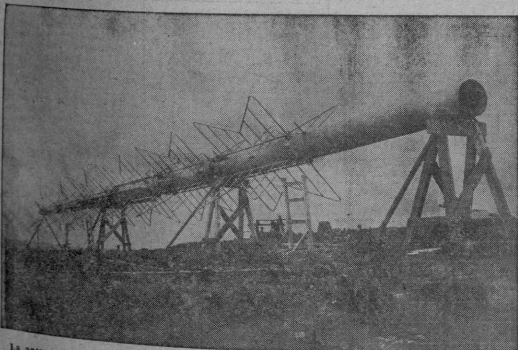
La antena de treinta metros de longitud que irá colocada en la torre de cuarenta metros de altura ya construida en la cima del Pedroso. Por tanto, la altura de la antena y su base de la Televisión de Santiago será de setenta metros. La fotografía fue realizada por Arturo durante un momento del montaje de los elementos que constituyen la antena.
