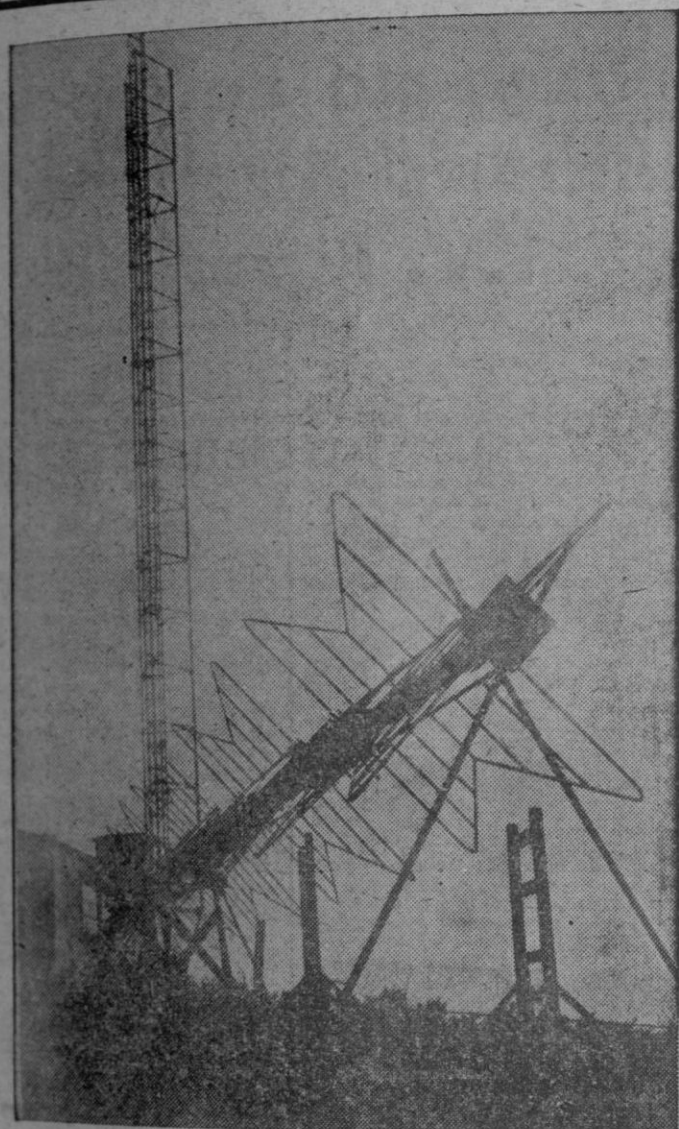
Vista de la antena de la TV santiagués y la torre en la que irá colocada. — (Foto Arturo)
