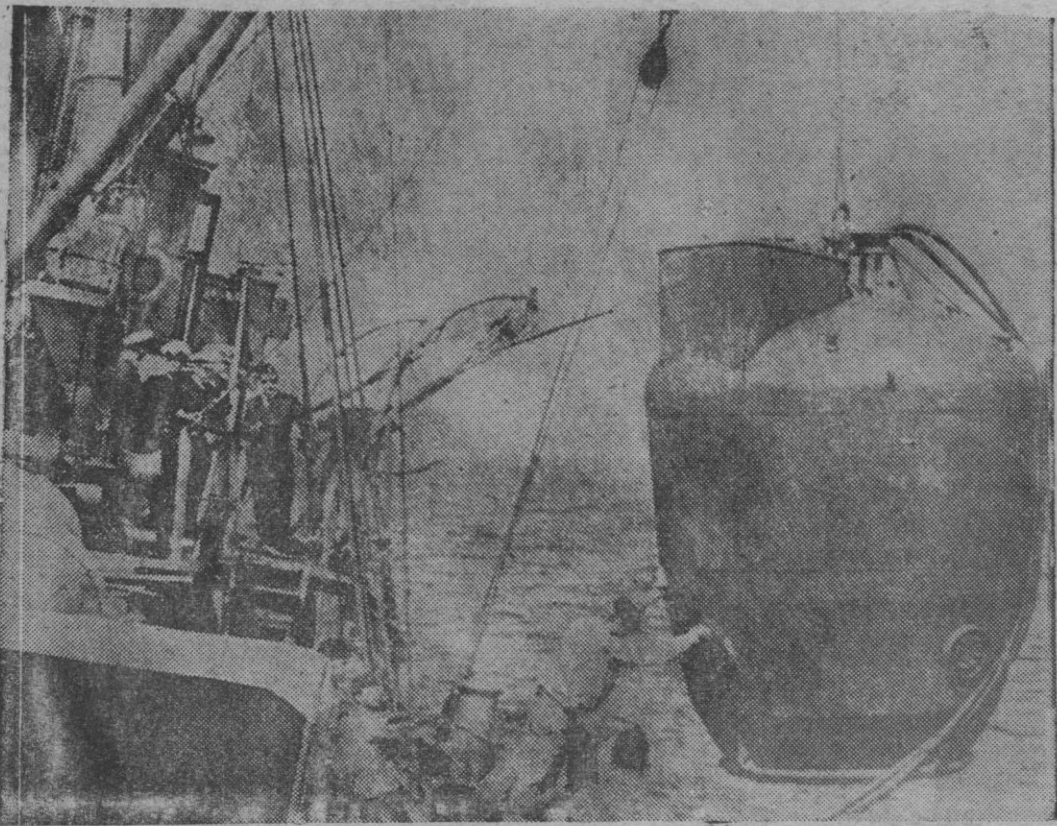
LUELSMINDE. En las costas de Jutlandia, oficiales de las Marinas sueca y danesa están probando en estos días un aparato de invención norteamericana para el salvamento de las tripulaciones de los submarinos hundidos. El depósito aquí fotografiado, que, dirigido por un hombre, desciende hasta la escotilla del sumergible, tiene capacidad para subir a siete hombres en cada viaje hasta la superficie.
