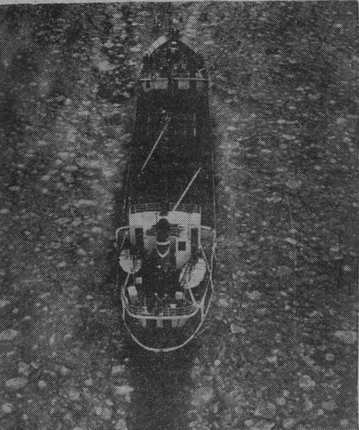
Con grandes dificultades este buque de carga se abre paso a través del hielo movedizo en el Canal de Kiel
