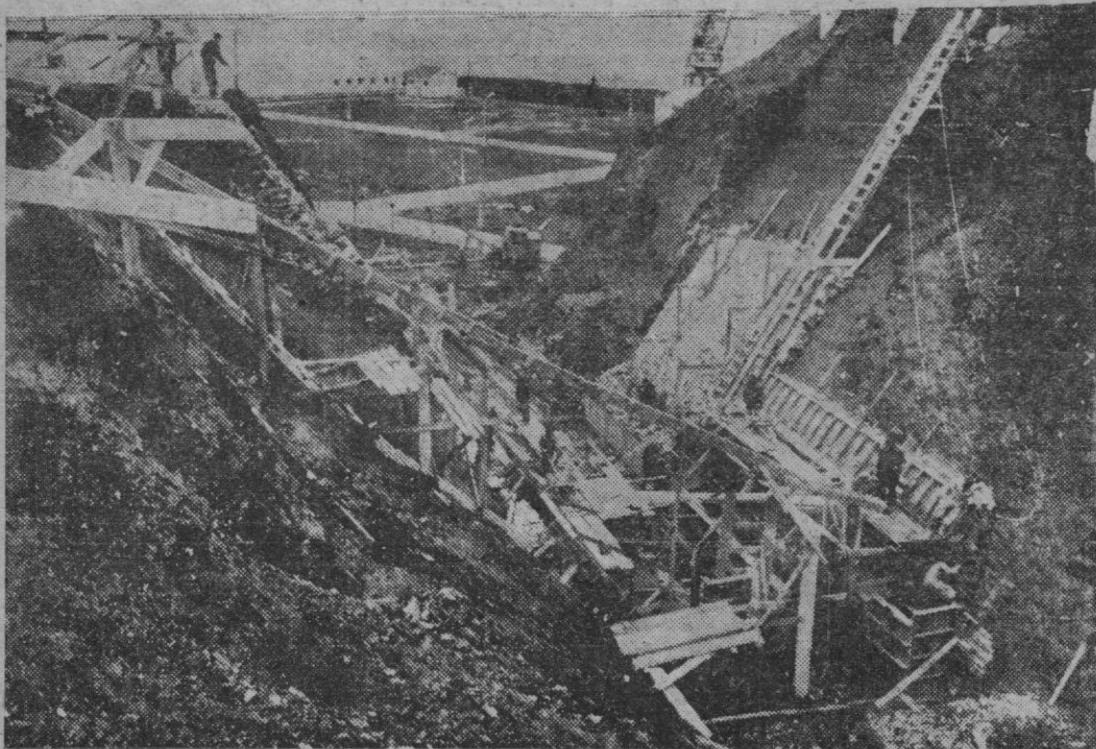
Las obras del cargadero de mineral de hierro (Foto ARJO)
