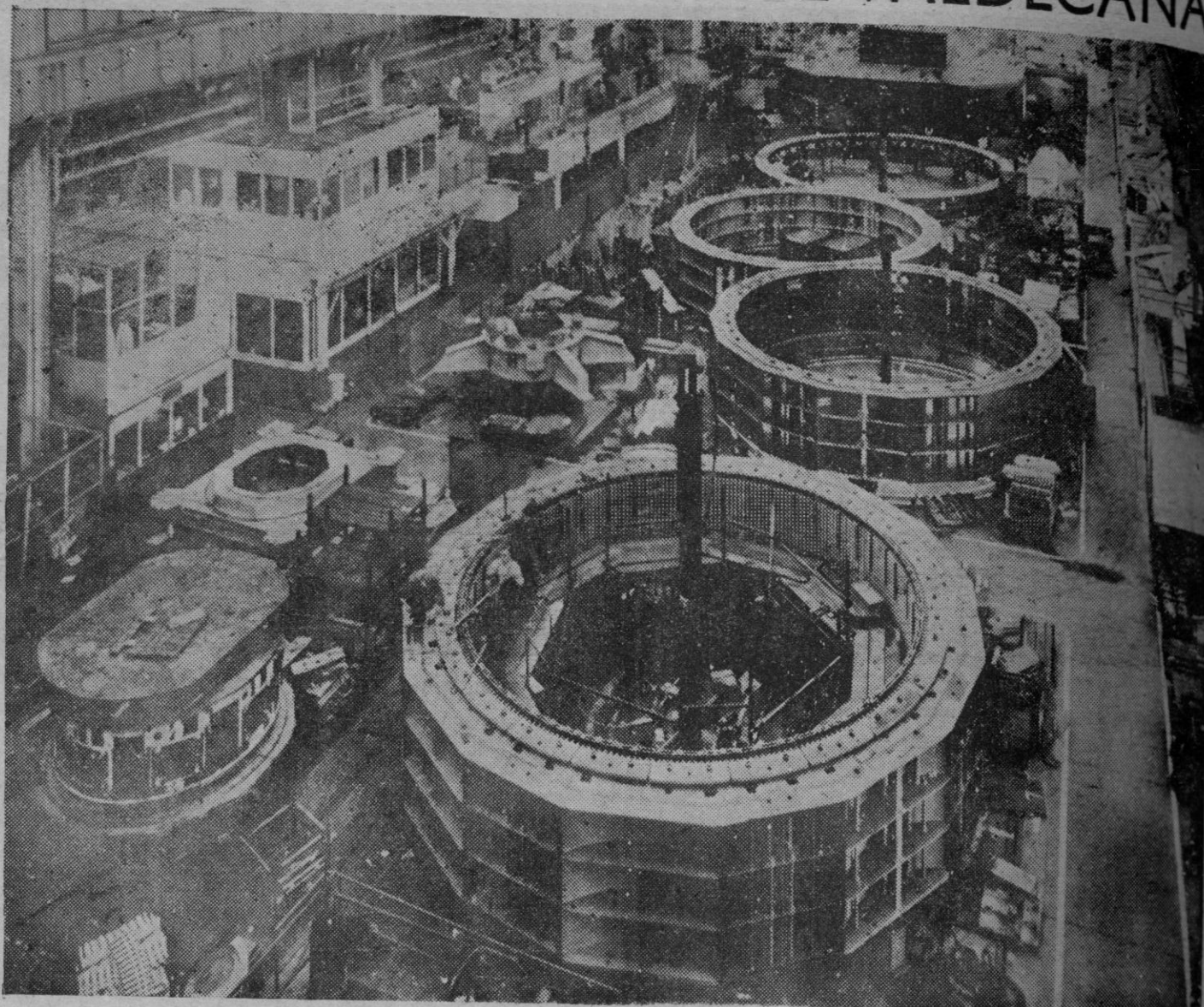
En primer plano, el estator de un generador para Valdecañas.
