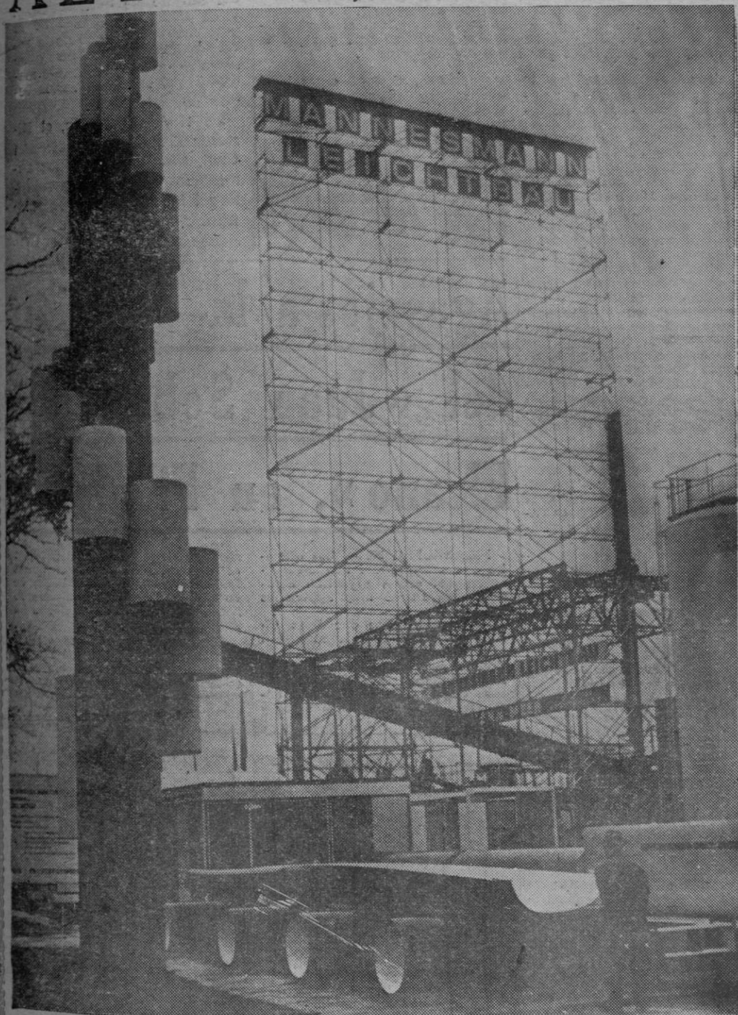
Quince pisos de altura tiene este andamiaje de erección rápida de la firma Mannesmann. El disco de andamiaje, dispuesto de modo completamente aislado, se aseguró mediante cables contra ráfagas. Figuró en la XVII Feria de Hannover, el escaparate del mundo industrial, a la que concurrieron 27 naciones.—(Foto D.A.D.)
