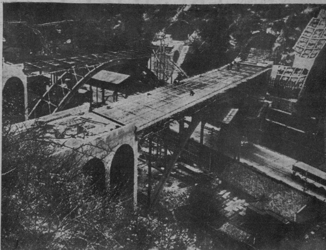
En la fotografía vemos el túnel de Torimoto, perteneciente a la carretera de tráfico rápido que se está construyendo entre Nagoya y Kobe. Esta carretera será de peaje es decir que los que la utilicen tendrán que pagar una cantidad, igual que para atravesar el túnel del Guadarrama. (Fotofiel)
