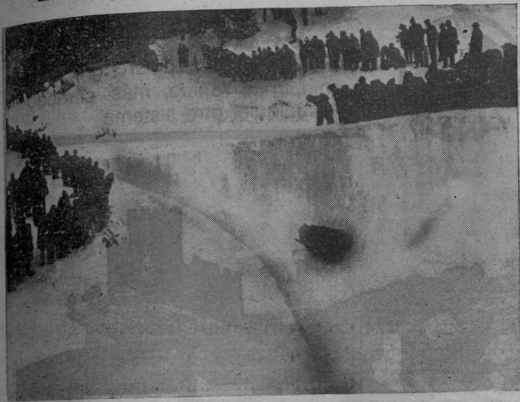
Pista olímpica de bobs. Es la más rápida del mundo y ha sido construida al pie de las montañas de Patscherkofel. Sus datos técnicos son: longitud 1.508 metros; diferencia de altura 141,50 metros; declive medio 9,43 por ciento; declive máximo 14 por ciento; número de vueltas, doce. (Foto EUROPA PRESS).
